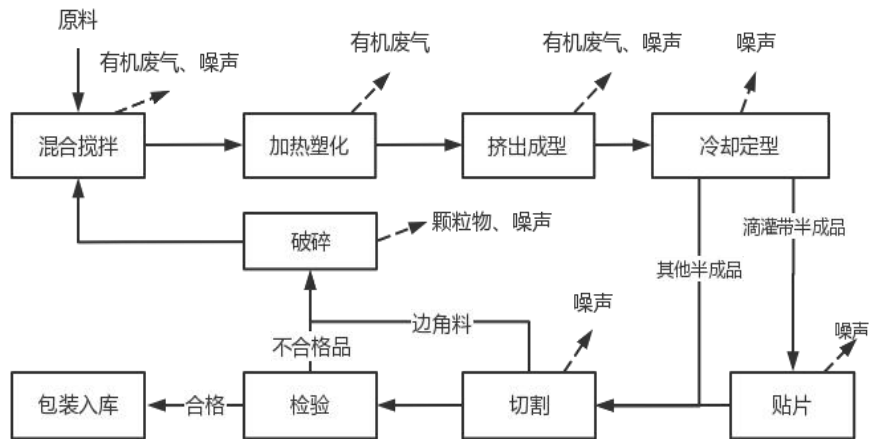
图 2-2 工艺流程及产污环节
