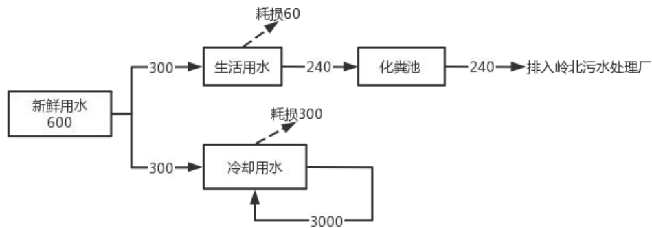
图 2-1 水平衡图 (m 3 /a)
