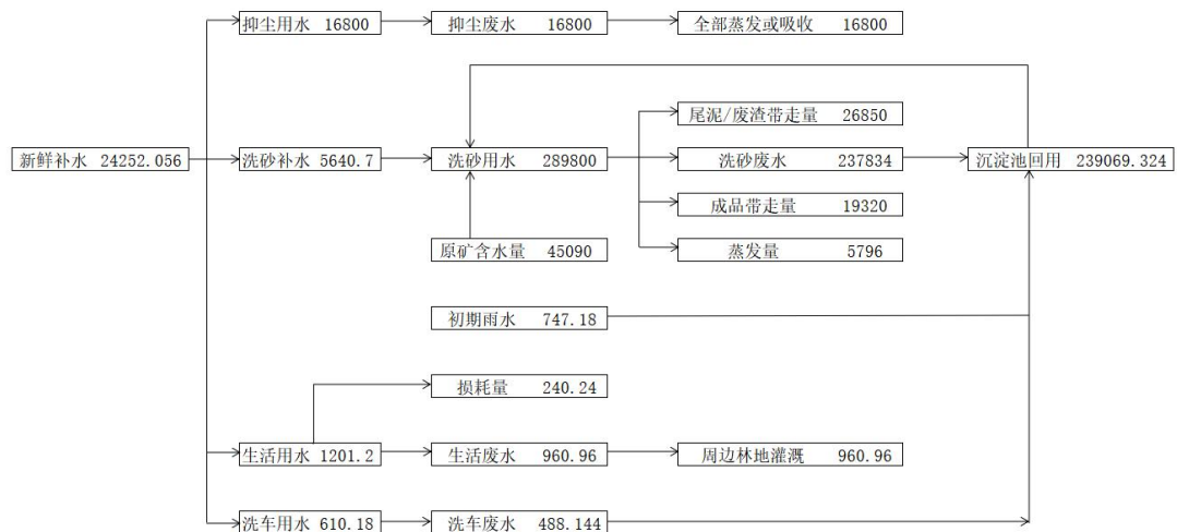
图2-3 项目水平衡图 单位: m 3 /a
