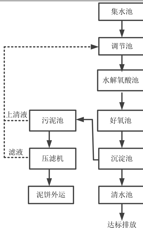
图3 自建废水处理站废水处理工艺流程图
