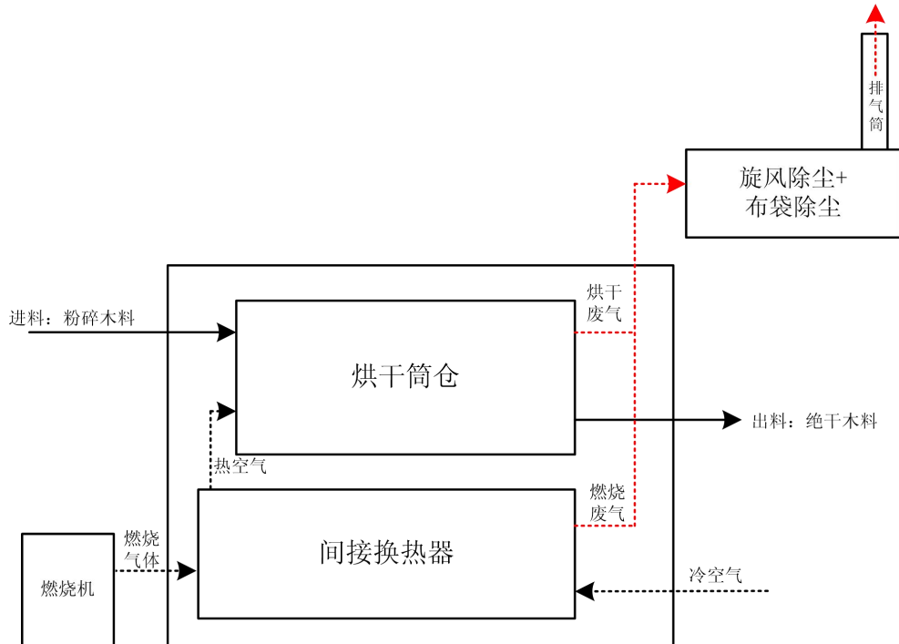
图 4-1 烘干工序设备情况示意图
