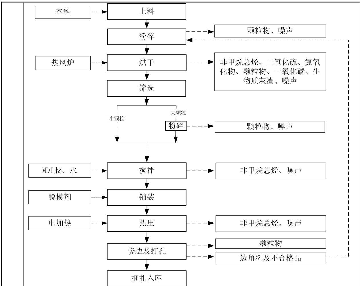
图 2-4 运营期生产工艺流程图
