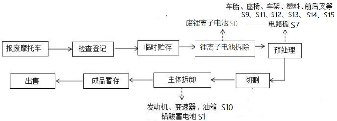
图 3 电动摩托车拆解
