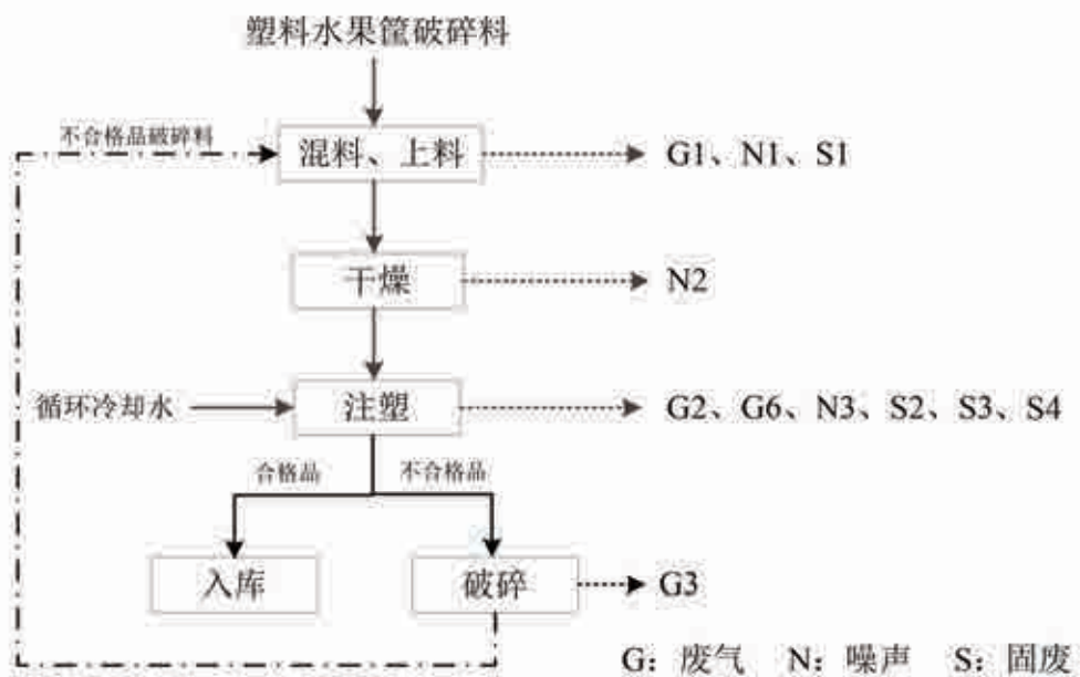
图3 塑料水果筐生产工艺及产污环节图
