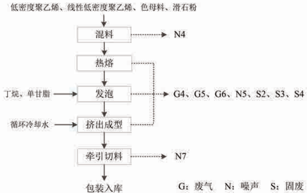
图6 水果发泡网套生产工艺及产污环节图
