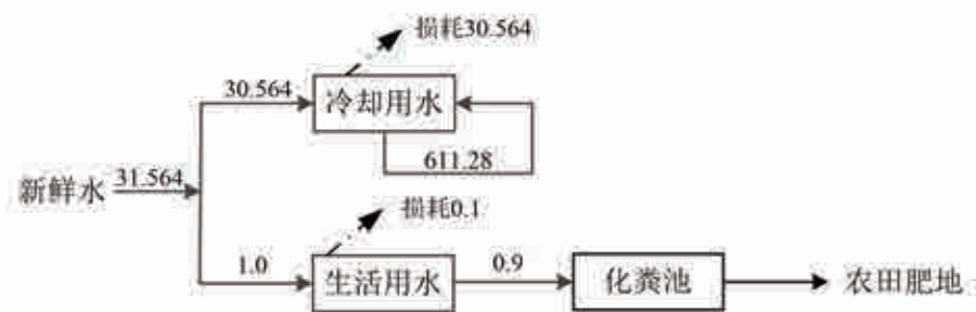
图 1 项目水平衡图 单位：m 3 /d
