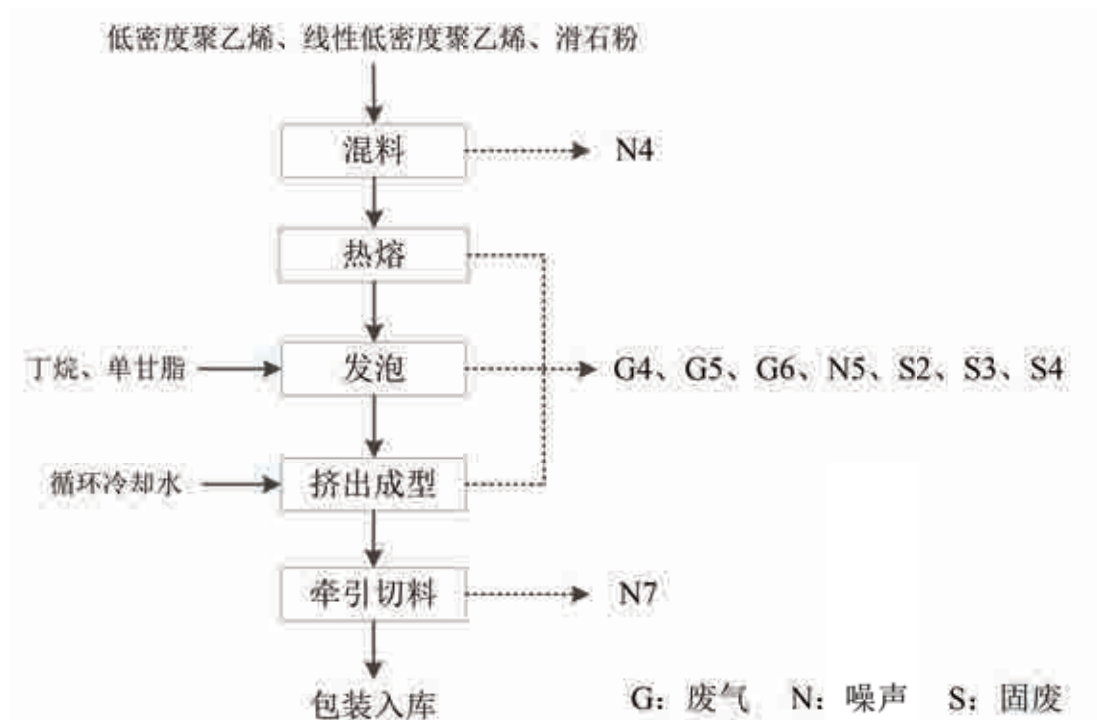
图5 水果发泡网垫生产工艺及产污环节图
