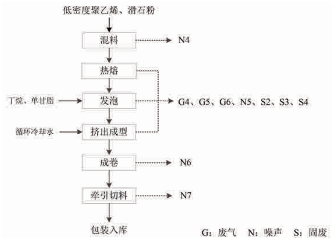
图 4 水果珍珠棉垫生产工艺及产污环节图
